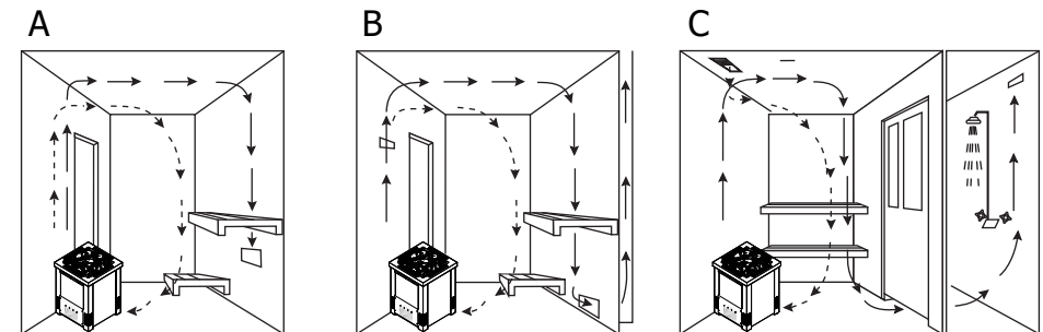
Kuva 4 | Saunahuoneen ilmanvaihto Fig. 4 | Sauna room ventilation
