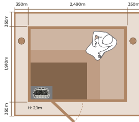
2121LL INT. VOL.: 7.34 m 3 SCA 8.0 kW
