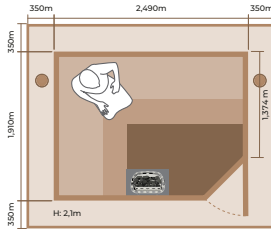
2121RLC INT. VOL.: 7.34 m 3 SCA 8.0 kW
