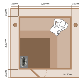
2323LL INT. VOL.: 8.85 m 3 SCA 9.0 kW
