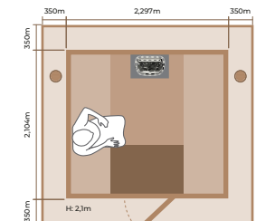
2125MD INT. VOL.: 8.06 m 3 SCA 8.0 kW
