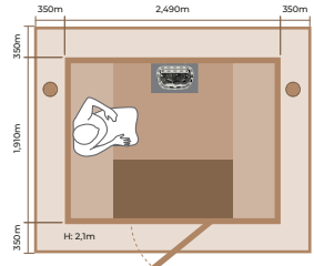
2121MD INT. VOL.: 7.34 m 3 SCA 8.0 kW
