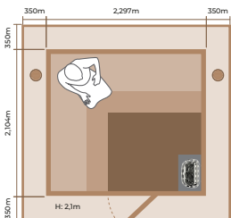
2125RL INT. VOL.: 8.06 m 3 SCA 8.0 kW
