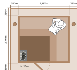
2125LL INT. VOL.: 8.06 m 3 SCA 8.0 kW
