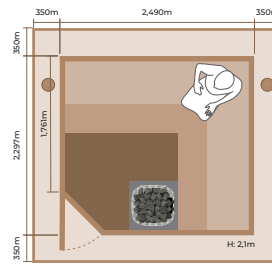
2325LLC INT. VOL.: 9.68 m 3 SAV 10.5 kW
