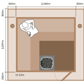
2325RL INT. VOL.: 9.68 m 3 SAV 10.5 kW
