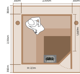
2123RLC INT. VOL.: 8.06 m 3 SCA 8.0 kW
