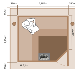
2125RLC INT. VOL.: 8.06 m 3 SCA 8.0 kW
