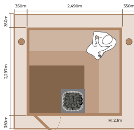
2325LL INT. VOL.: 9.68 m 3 SAV 10.5 kW
