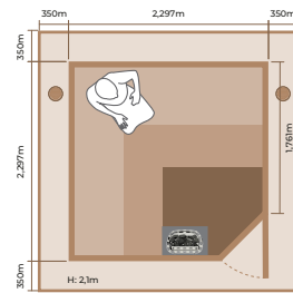
2323RLC INT. VOL.: 8.64 m 3 SCA 9.0 kW
