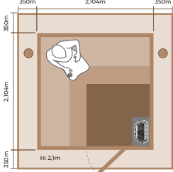
2123RL INT. VOL.: 8.06 m 3 SCA 8.0 kW
