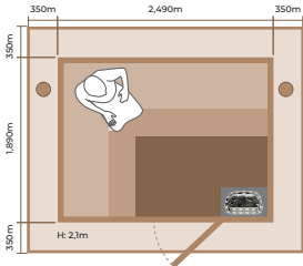
2121RL INT. VOL.: 7.34 m 3 SCA 8.0 kW
