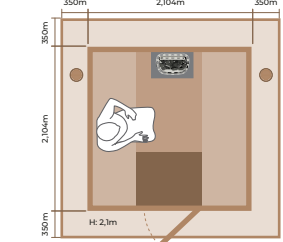
2123MD INT. VOL.: 8.06 m 3 SCA 8.0 kW
