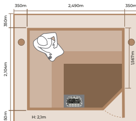
2323RLC INT. VOL.: 8.64 m 3 SCA 9.0 kW
