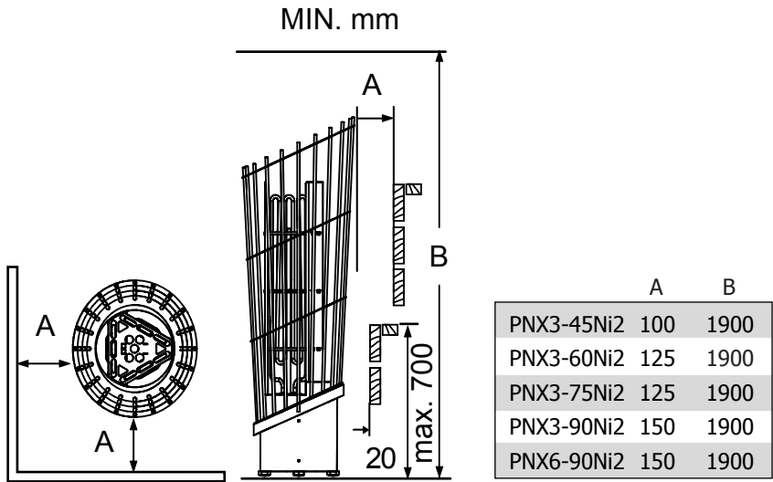
Kuva 2 | Minimisuojaetäisyydet (mm) Fig. 2 | Minimum safety distances (mm)
