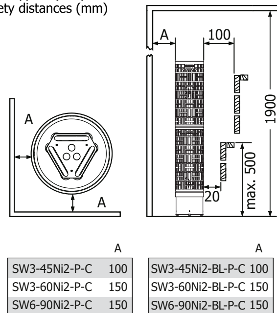
Kuva 2 Minimisuojaetäisyydet (mm) Fig. 2 Minimum safety distances (mm)
