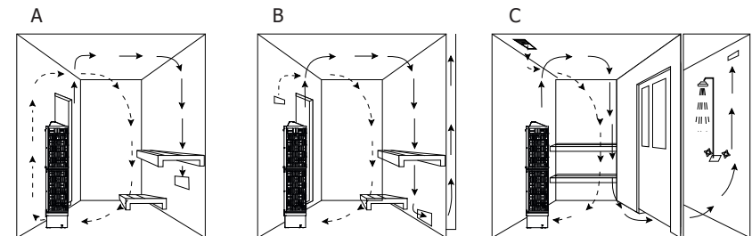
Kuva 7 Ilmanvaihto Fig. 7 Air ventilation
