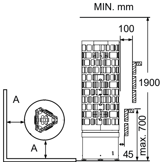
Kuva 2 Fig. 2 Minimisuojaetäisyydet (mm) Minimum safety distances (mm)
