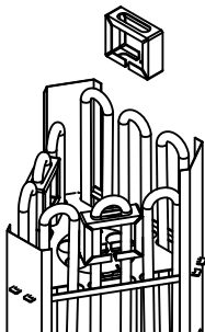
Kuva 4 Fig. 4 Vastuspidikkeet Heating Element Separator
