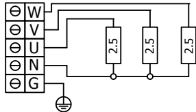
ARI3-75NS-WL 7,5 kW
