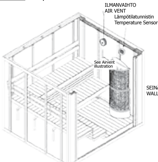
Kuva 6 | Lämpötilatunnistimen sijainti Fig. 6 | Temperature Sensor Location
