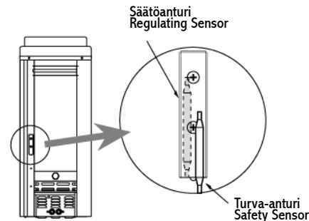
Kuva 7 Anturien sijainnit Fig. 7 Sensor Location
