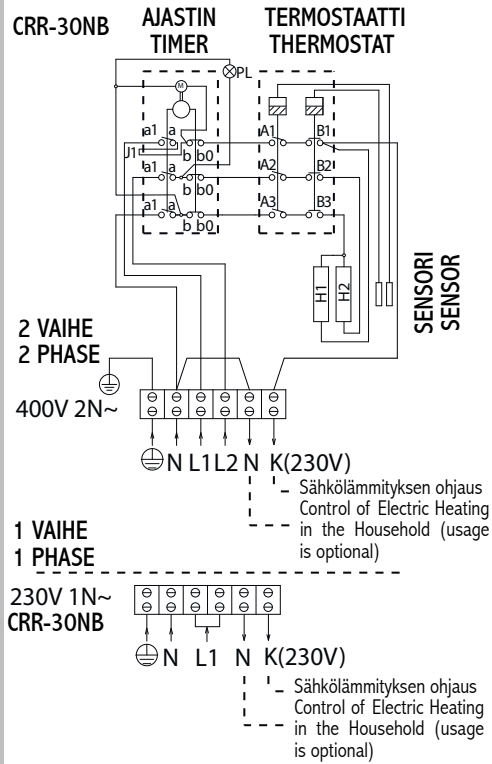
Kuva 5 Kytentäkaavio Fig. 5 Electrical Diagram
