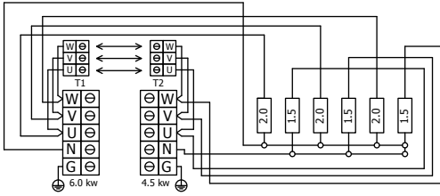
DRFT6-105NS 10,5 kW
