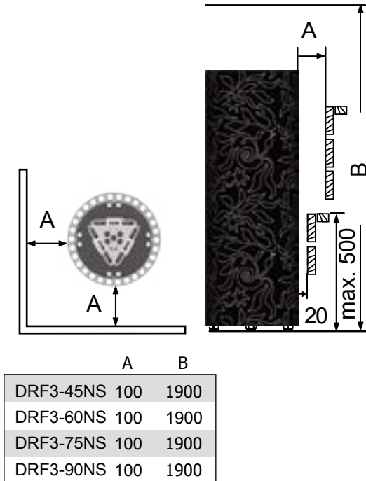
Kuva 2 | Vähimmäisetäisyydet (mm) Fig. 2 | Minimum safety distances (mm)
